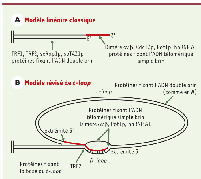
Figure 3. Modèles de structure des télomères. A. Modèle classique d'une extrémité chromosomique avec une courte extension en 3' (en rouge) et un complexe protéique protégeant l'ADN chromosomique (modèle linéaire). B. Les télomères des mammifères se terminent par de larges boucles, les t-loops (telomere loops). Le double brin télomérique se replie sur lui-même, l'extension 3' simple brin s'insère dans la portion double brin et engendre la D-loop (displacement loop). La protéine TRF2 se fixe à la base du D-loop in vitro . Les t-loops , en association avec un complexe protéique terminal, pourraient permettre de différencier les extrémités des chromosomes des cassures double brin dans l'ADN, et éviter ainsi la détection des télomères par la machinerie de réparation des cassures d'ADN. Les régions simple brin du t-loop et les extensions en 3' sont indiquées en rouge. TRF1, 2: telomeric repeat binding factor 1, 2 ; scRap1p: protéine télomérique RAPI de Saccharomyces cerevisiae ; Cdc13p: telomere binding protein Cdc13p ; Pot1p: protection of telomeres 1 ; hnRNP A1: heterogeneous ribonucleoprotein A1 .
